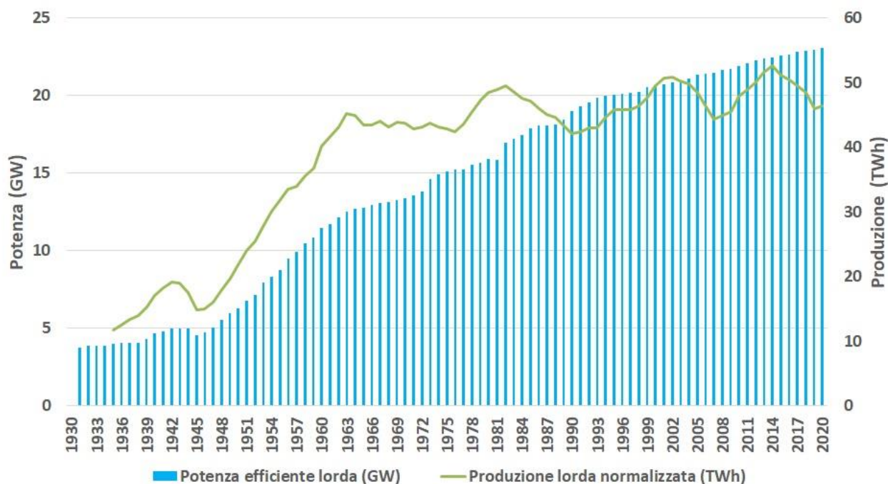
Fig. 20 – Produzione di energia idroelettrica e capacità installata in Italia (Fonte: SNPA, 2021 209 )
