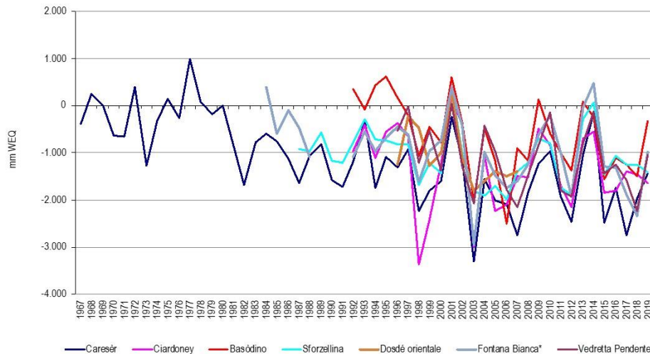
Fig. 10 – Bilancio di massa netto di alcuni ghiacciai italiani (Fonte: SNPA, 21/2021 38 )
